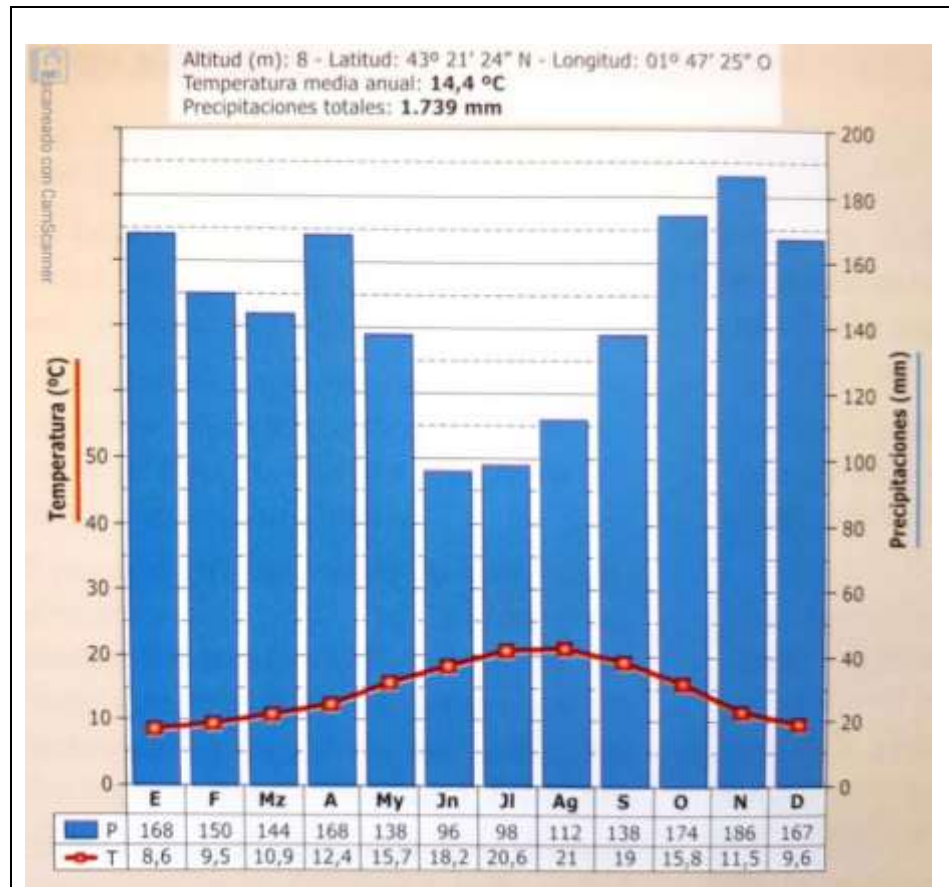
Imagen nº 1. Climograma.
